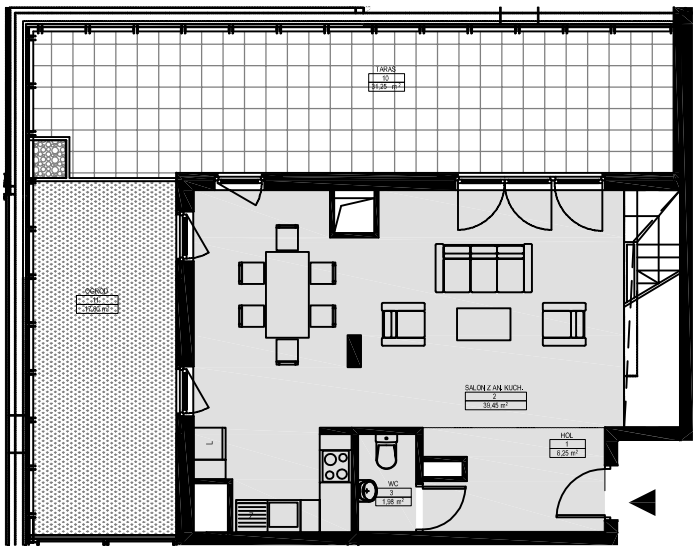
POZIOM 1
