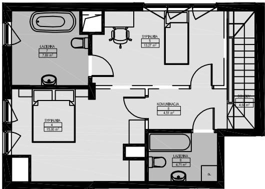
POZIOM 2
